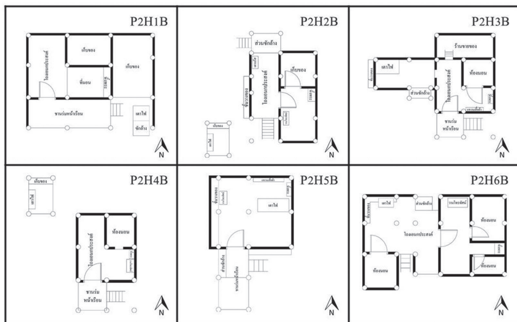
ภาพที่ 15 พื้นที่การใช้งานภายในเรือนกะเหรี่ยงโปว์แบบผสมผสานดั้งเดิมบ้านหนองปู
