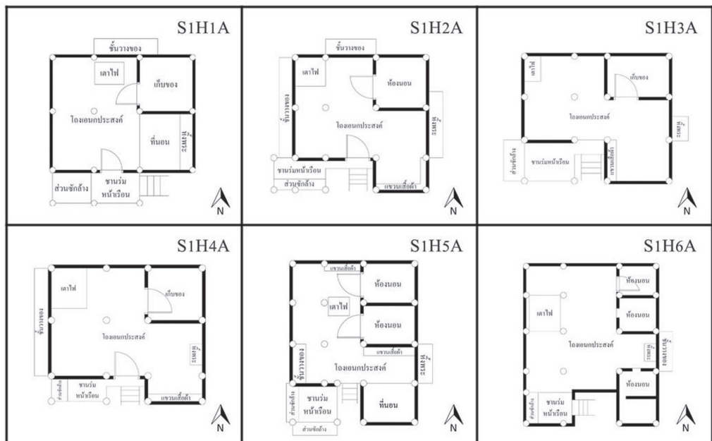
ภาพที่ 12 พื้นที่การใช้งานภายในเรือนกะเหรี่ยงสะกอแบบดั้งเดิมบ้านศรีเวียงชัย
