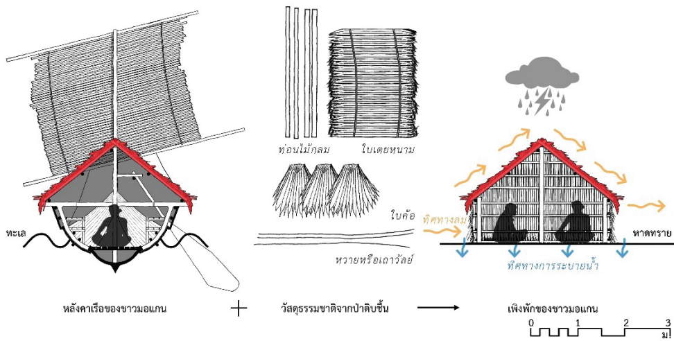
ภาพที่ 9 การก่อรูปของเพิงพักของชาวมอแกน
