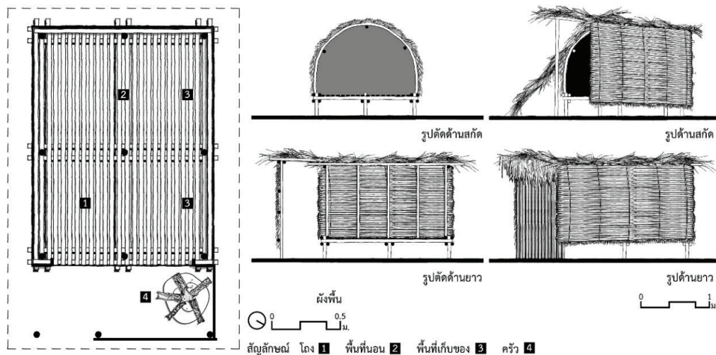
ภาพที่ 7 การจัดวางพื้นที่ใช้สอยภายในเพิงพักของชาวอุรักลาไวย์
