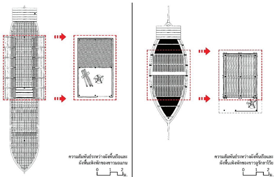
ภาพที่ 8 ซ้าย : ความสัมพันธ์ระหว่างผืนพื้นเรือและผืนเพิงพักของชาวมอแกน ขวา : ความสัมพันธ์ระหว่างผืนพื้นเรือและผืนเพิงพักของชาวอุรักลาโว้ย
