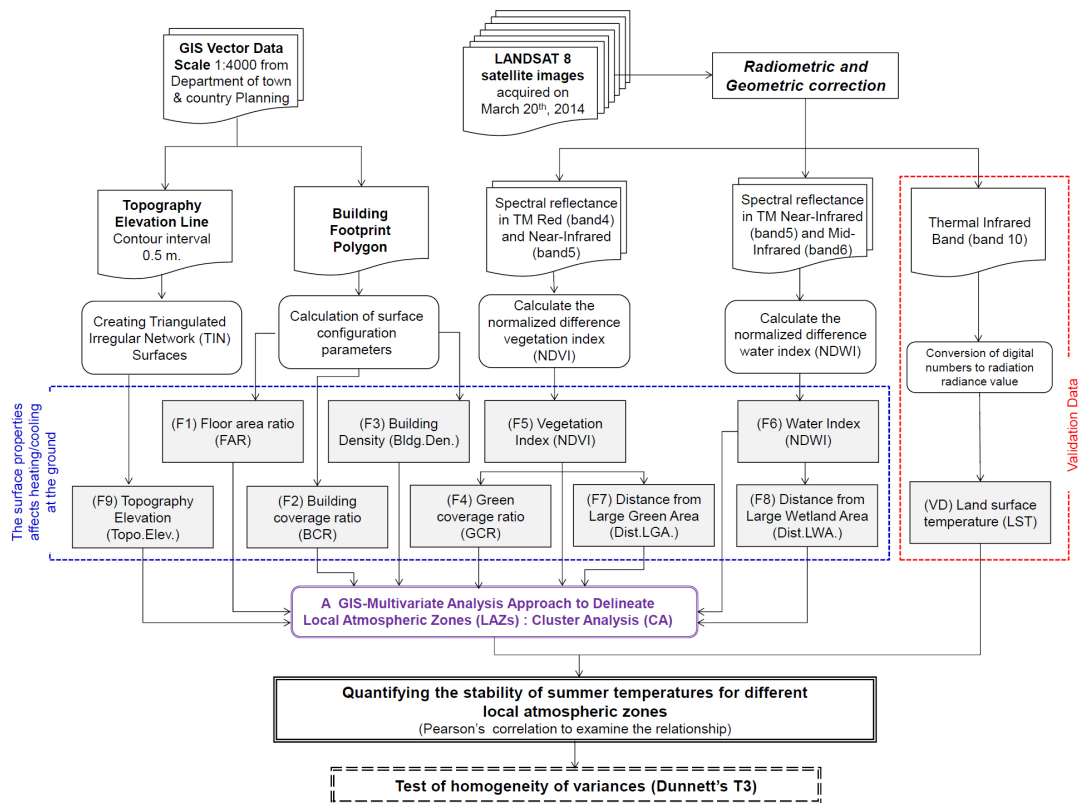
รูปที่ 3 ขั้นตอนการจำแนกเขตบรรยากาศประจำถิ่น (Methods for local atmospheric zones classification) ในฤดูร้อนเมืองเชียงใหม่ ที่มา: ผู้วิจัย
