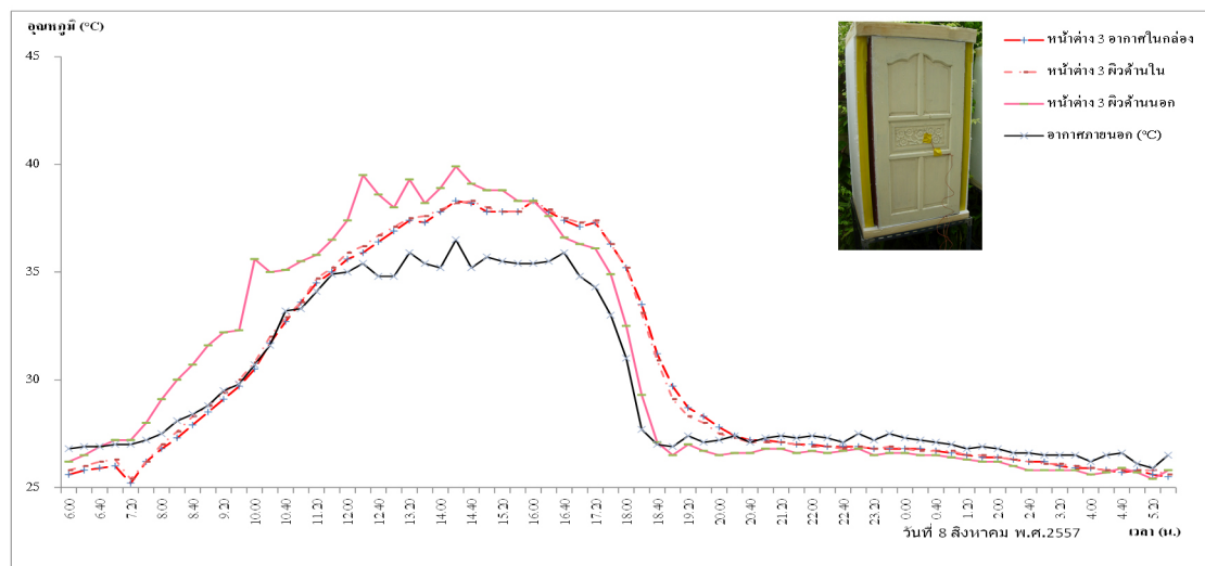
รูปที่ 20 อุณหภูมิของหน้าต่างแบบที่ 3 ด้านทิศใต้
