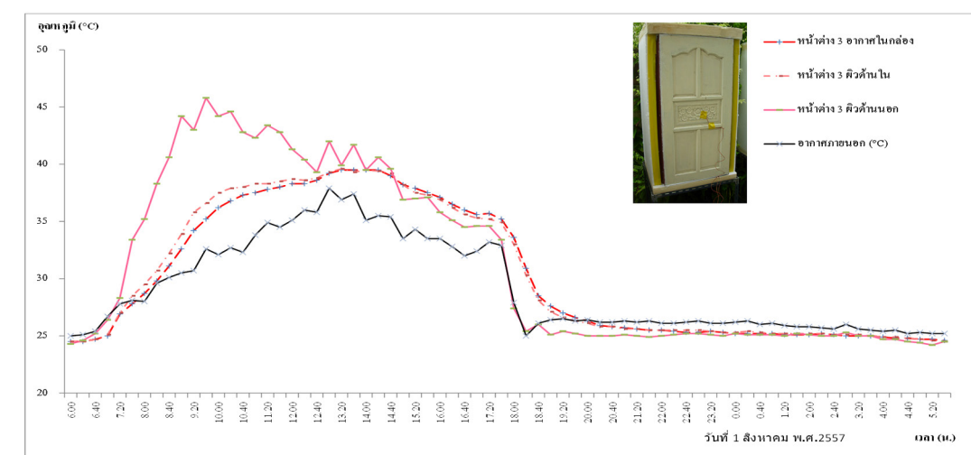
รูปที่ 10 อุณหภูมิของหน้าต่างแบบที่ 3 ด้านทิศตะวันออก
