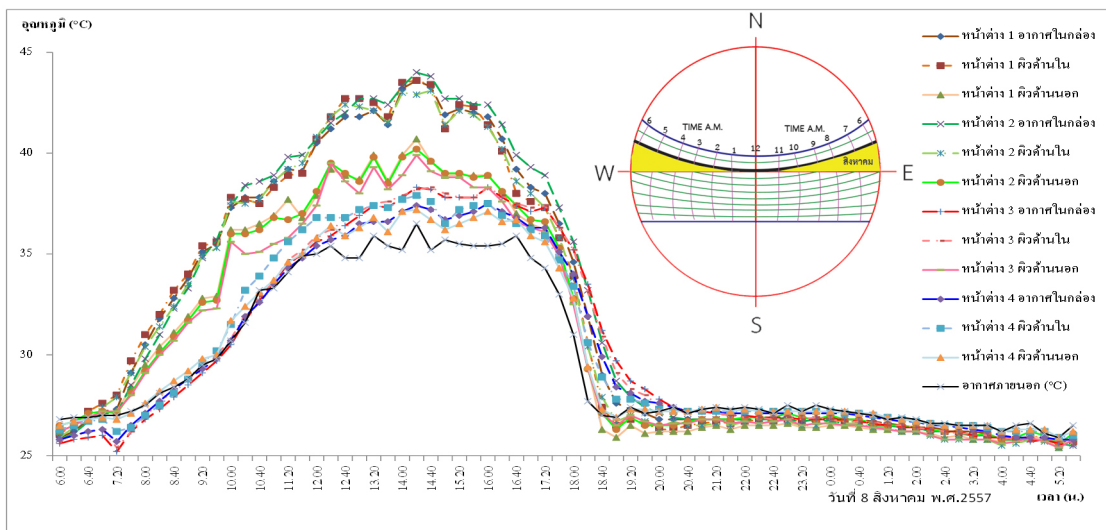
รูปที่ 17 อุณหภูมิของหน้าต่างแบบที่ 1-4 ด้านทิศใต้
