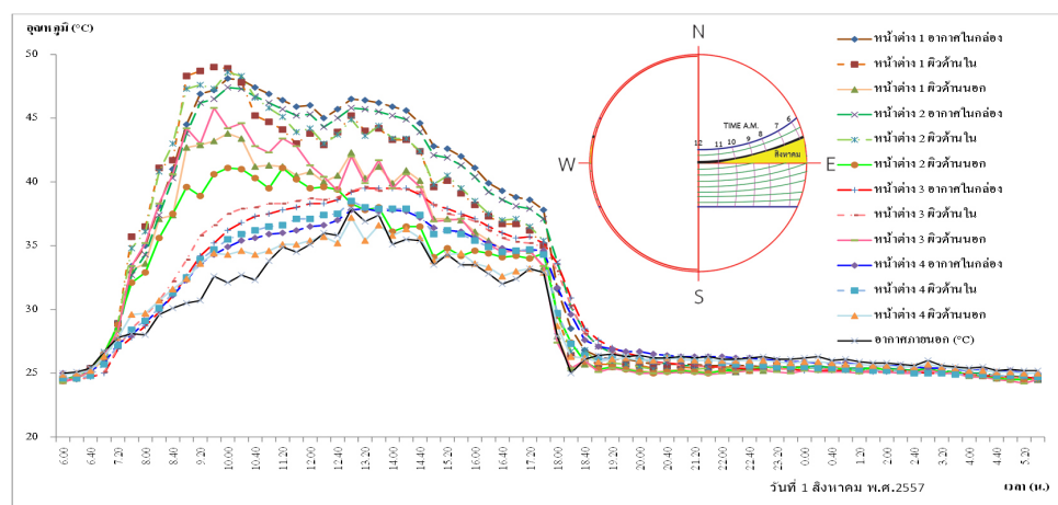
รูปที่ 7 อุณหภูมิของหน้าต่างแบบที่ 1-4 ด้านทิศตะวันออก
