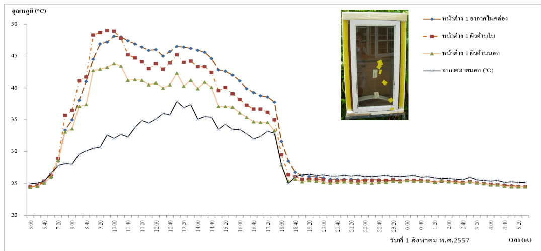
รูปที่ 8 อุณหภูมิของหน้าต่างแบบที่ 1 ด้านทิศตะวันออก
