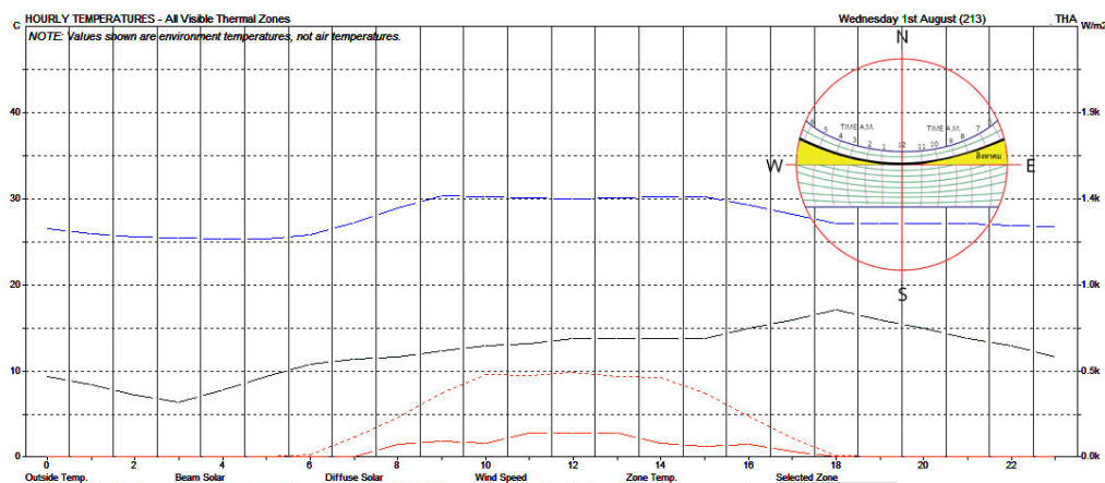
รูปที่ 6 การวิเคราะห์อุณหภูมิเฉลี่ยในแต่ละชั่วโมงของวันในเดือนสิงหาคม
