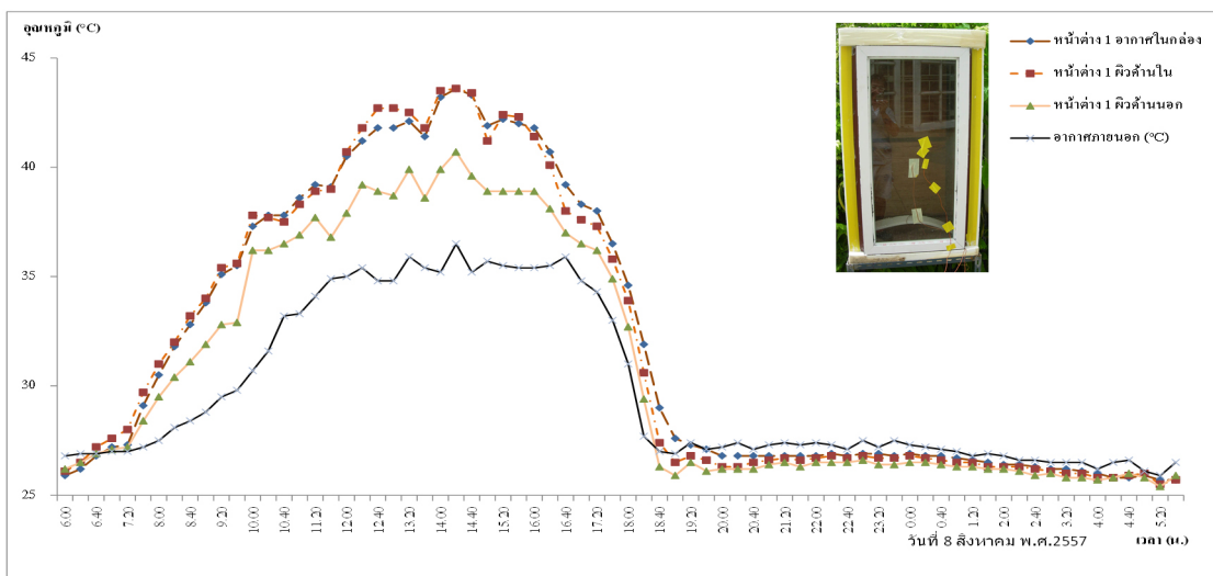
รูปที่ 18 อุณหภูมิของหน้าต่างแบบที่ 1 ด้านทิศใต้
