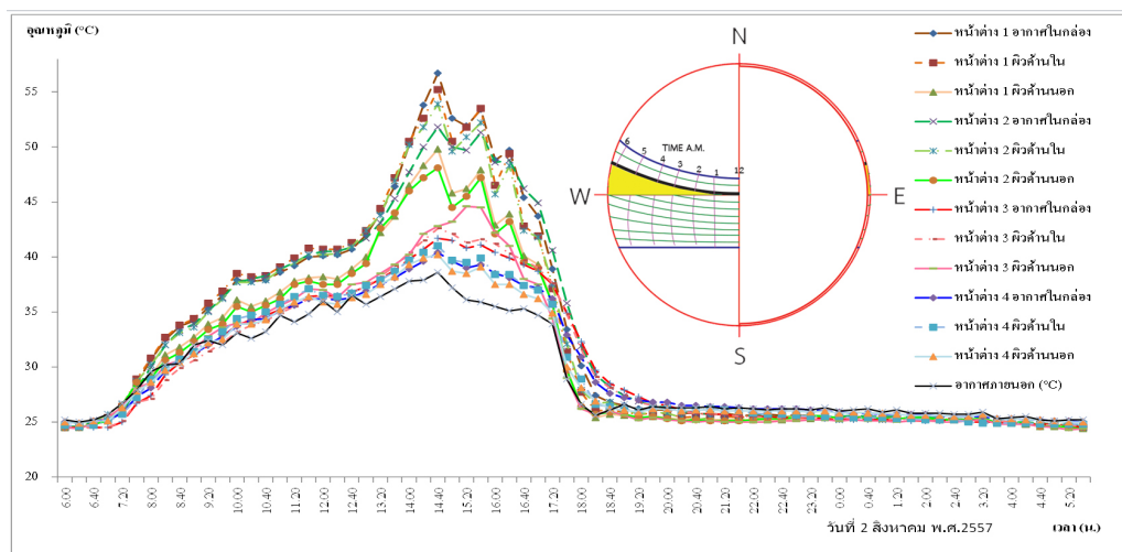
รูปที่ 12 อุณหภูมิของหน้าต่างแบบที่ 1-4 ด้านทิศตะวันตก
