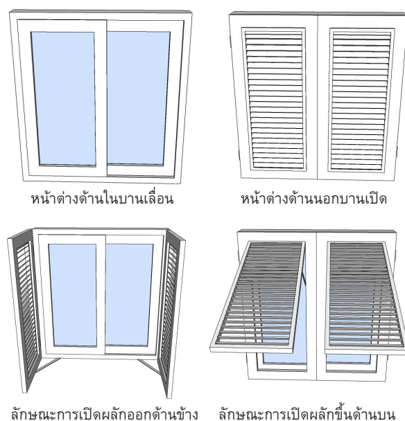
รูปที่ 2 ลักษณะหน้าต่างสองชั้นที่ทำการออกแบบ
