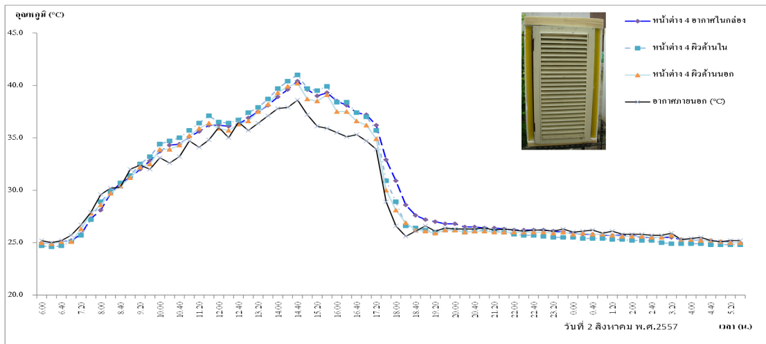
รูปที่ 16 อุณหภูมิของหน้าต่างแบบที่ 4 ด้านทิศตะวันตก
