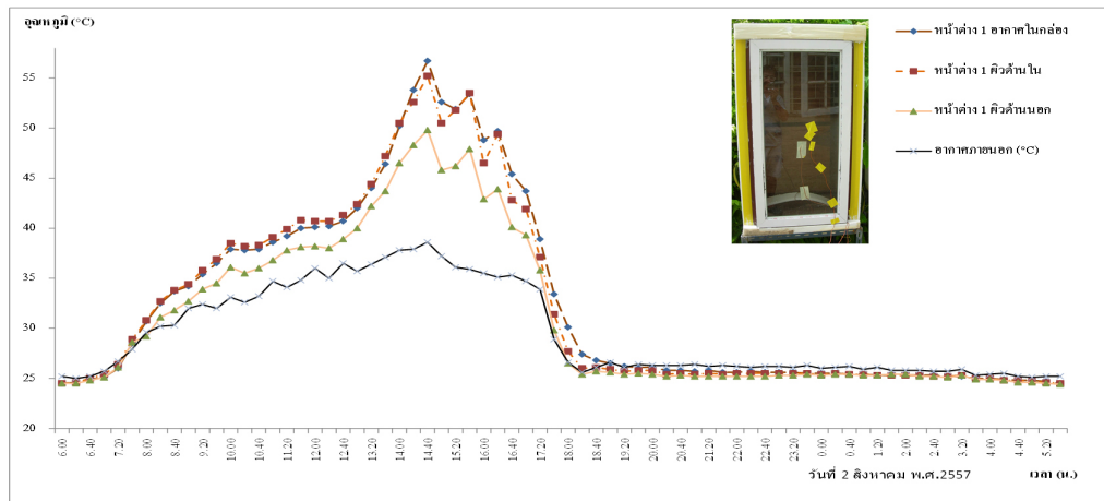
รูปที่ 13 อุณหภูมิของหน้าต่างแบบที่ 1 ด้านทิศตะวันตก
