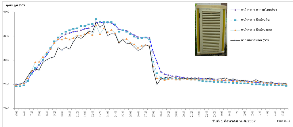
รูปที่ 11 อุณหภูมิของหน้าต่างแบบที่ 4 ด้านทิศตะวันออก
