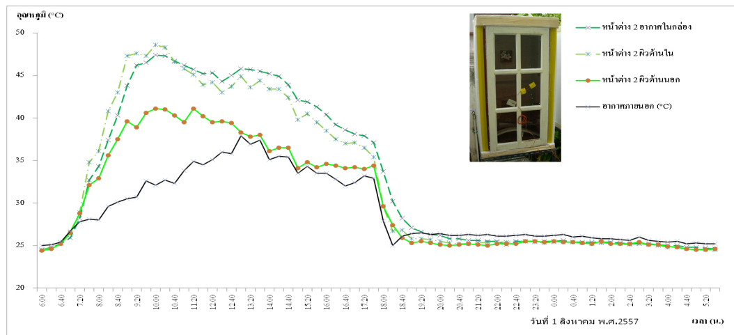
รูปที่ 9 อุณหภูมิของหน้าต่างแบบที่ 2 ด้านทิศตะวันออก
