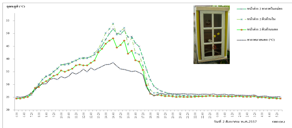
รูปที่ 14 อุณหภูมิของหน้าต่างแบบที่ 2 ด้านทิศตะวันตก
