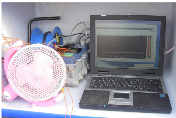
รูปที่ 5 ชุดเครื่องบันทึกข้อมูล (Data logger)
