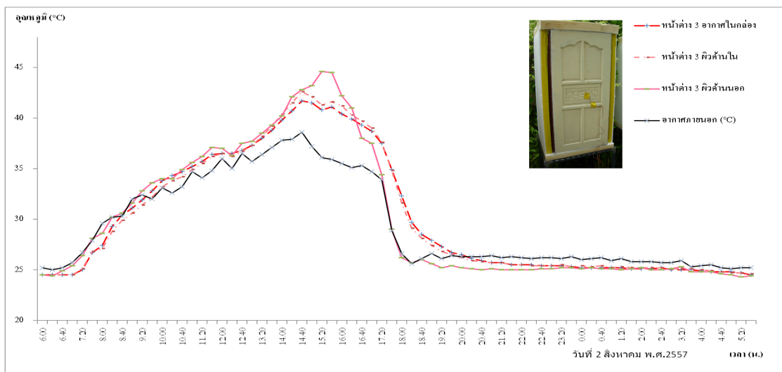
รูปที่ 15 อุณหภูมิของหน้าต่างแบบที่ 3 ด้านทิศตะวันตก
