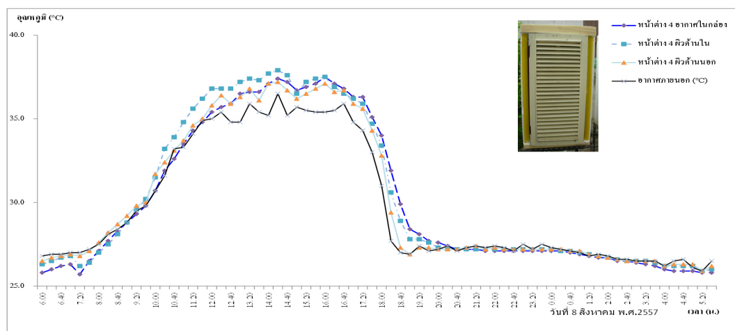
รูปที่ 21 อุณหภูมิของหน้าต่างแบบที่ 4 ด้านทิศใต้
