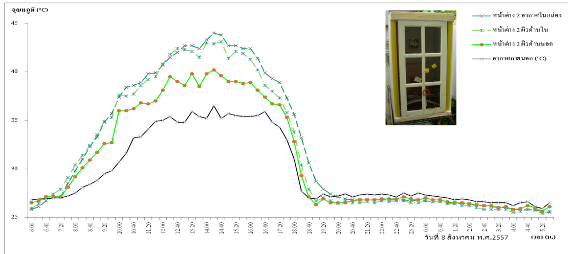
รูปที่ 19 อุณหภูมิของหน้าต่างแบบที่ 2 ด้านทิศใต้
