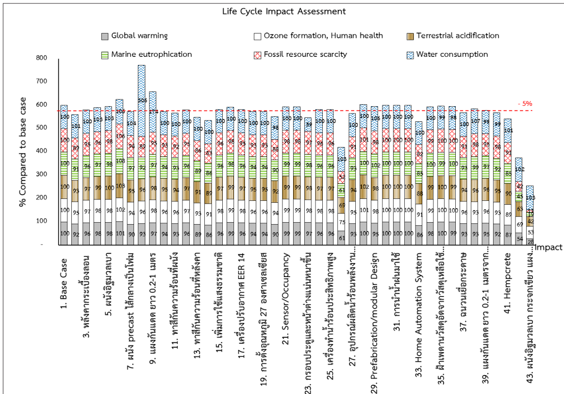
รูปที่ 11 ผลการประเมินผลกระทบสิ่งแวดล้อมตลอดวัฏจักรชีวิตของบ้านทุกมาตรการ (Life cycle analysis of all measures applied to a detached house case study.)
