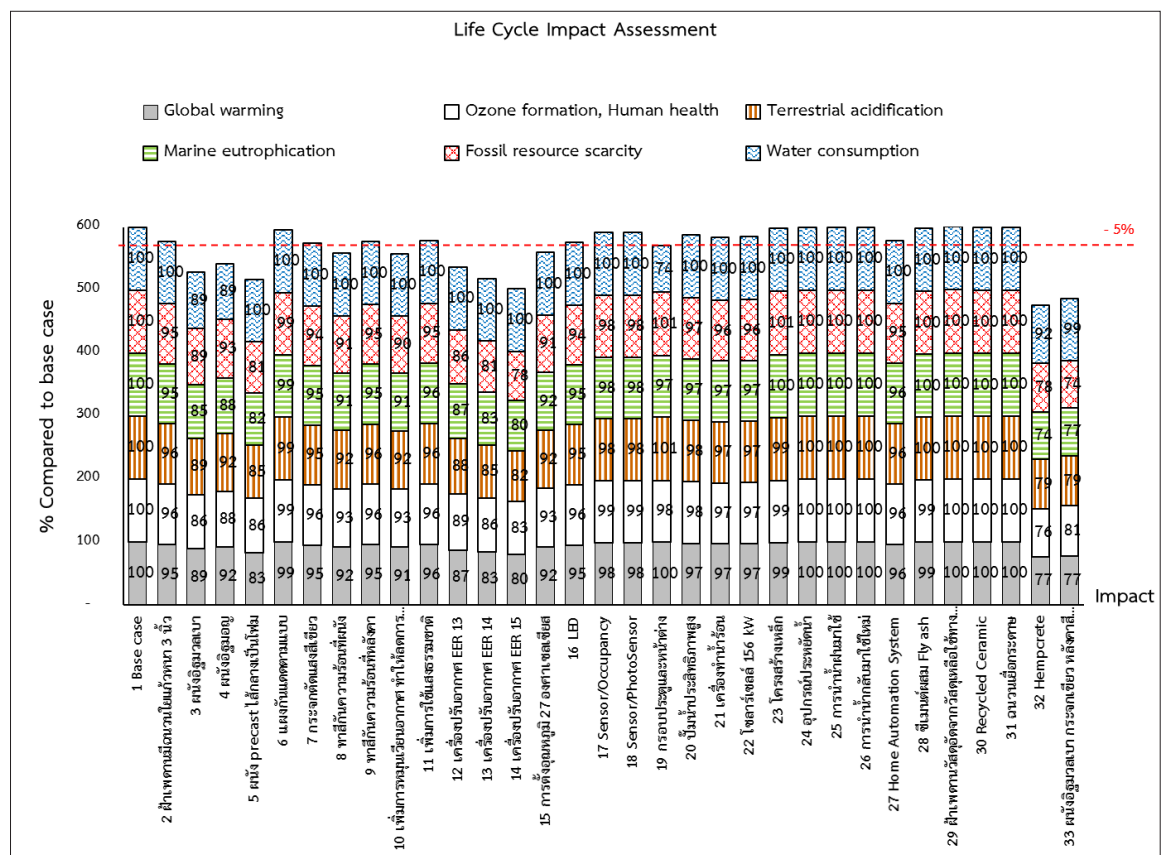
รูปที่ 12 ผลการประเมินผลกระทบสิ่งแวดล้อมตลอดวัฏจักรชีวิตของคอนโดมิเนียม ทุกมาตรการ (Life cycle analysis of all measures applied to a condominium case study.)
