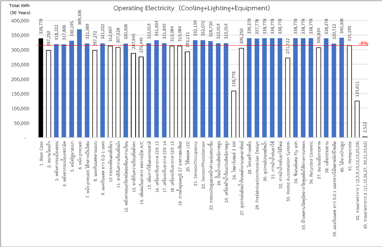
รูปที่ 8 ปริมาณการใช้ไฟฟ้าระหว่างการใช้งานของรูปแบบทางเลือกต่าง ๆ ของบ้านตลอดช่วงการใช้งาน 50 ปี (Fifty years operating electricity cost of each design option.)
