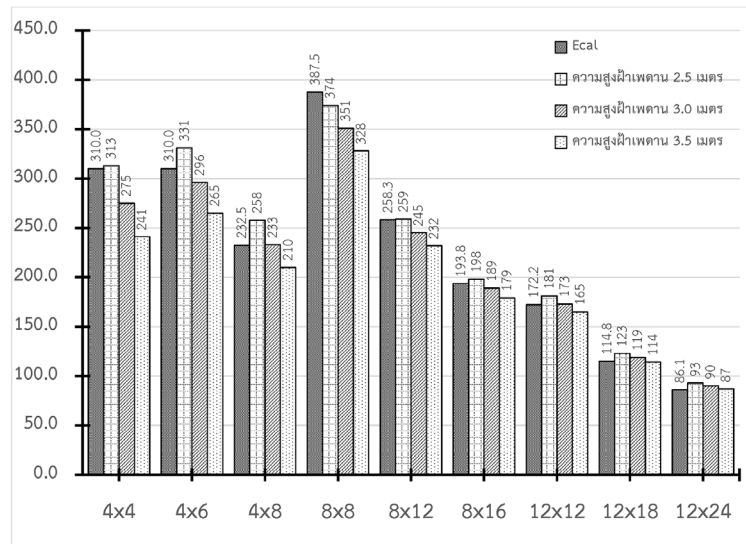
รูปที่ 17 เปรียบเทียบค่าความสว่างที่ได้จากสมการคำนวณแบบง่าย (Ecal) จากสมการที่ 7 และค่าที่คำนวณจากโปรแกรมคอมพิวเตอร์ (Esim) (Comparison calculated illuminance values (Ecal) by Equation 7 and computer simulated illuminance values (Esim))
