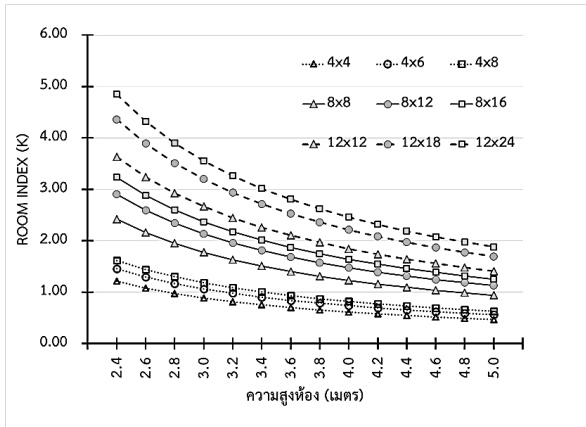
รูปที่ 9 ค่าดัชนีห้อง (K) ที่คำนวณได้สำหรับห้องที่มีขนาดและรูปร่างแตกต่าง (Calculated room index (K) for various room configurations.)
