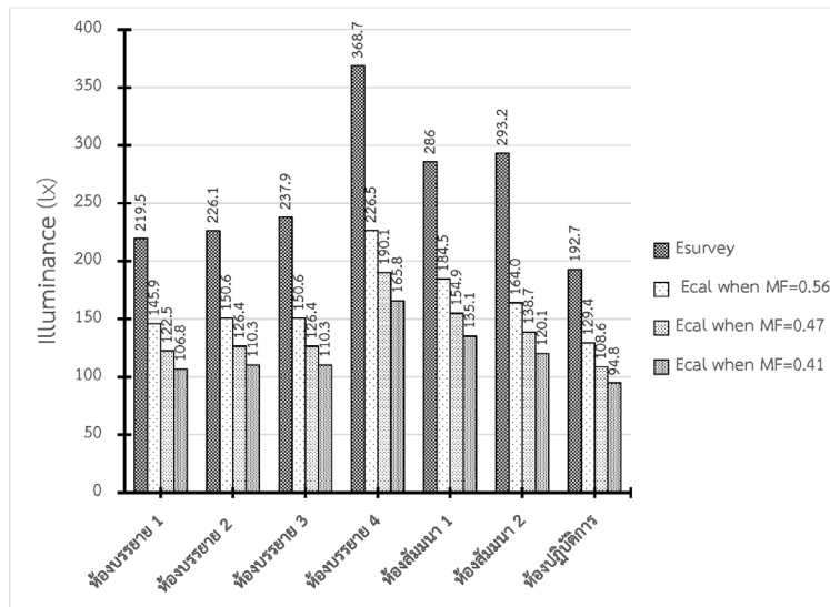
รูปที่ 15 ความสว่างเฉลี่ยจากการสำรวจและความสว่างที่คำนวณจากวิธีการลูเมน Averaged illuminance values from survey and calculated illuminance values by the lumen method.
