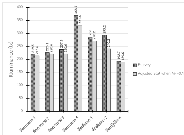
รูปที่ 16 ความสว่างเฉลี่ยจากการสำรวจและความสว่างที่ปรับค่าจากค่าที่ได้จากการคำนวณจากวิธีการลูเมน (Averaged illuminance values from survey and adjusted illuminance values from calculated illuminance values by the lumen method.)
