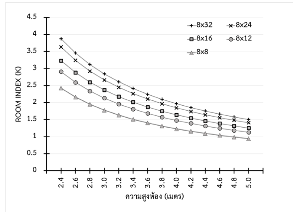
รูปที่ 10 ความสัมพันธ์ของค่า K ของห้องกว้าง 8 เมตรที่มีสัดส่วนแปลน 1:1 ถึง 1:4 (Relationships of the room index (K) values for rooms with 8 meter width, where room ratios are from 1:1 to 1:4)
