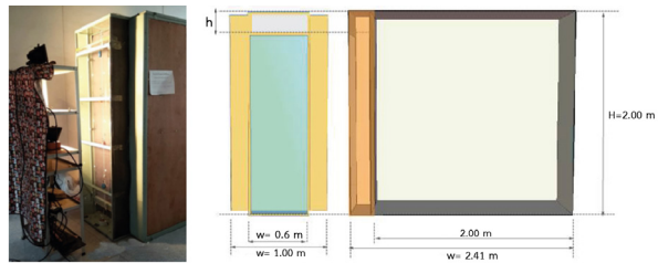
รูปที่ 1 ลักษณะของกล่องทดลอง (Characteristics of the experimental box)
