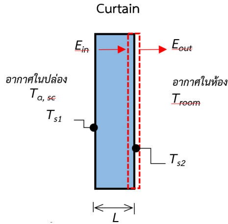
รูปที่ 7 แผนภาพการถ่ายเทความร้อนคงตัวผ่านม่านในงานวิจัยนี้ (The diagram of steady heat transfers through curtain in this research)
