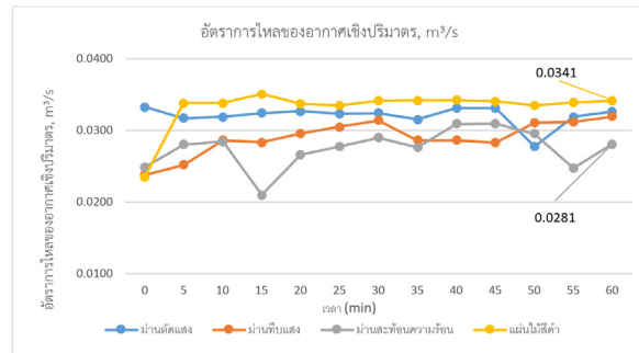
รูปที่ 6 อัตราการไหลของอากาศเชิงปริมาตร (Volumetric air flow rate)
