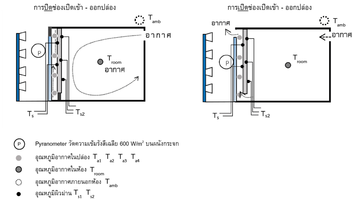
รูปที่ 2 การบันทึกข้อมูลในกล่องทดลอง (Data recording of experimental box)
