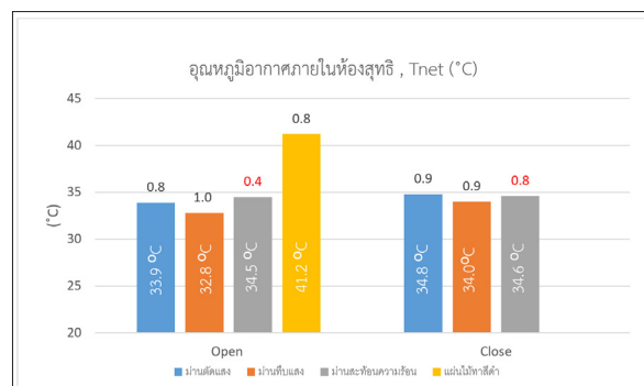
รูปที่ 8 การเปรียบเทียบอุณหภูมิอากาศภายในห้องสุทธิ ในกรณี เปิดและปิดช่องอากาศ ของม่านทั้ง 3 ชนิดและแผ่นไม้ทาสีดำ (The net room air temperature comparison in the case of opening and closing ventilation chimney of all 3 types of sheet)
