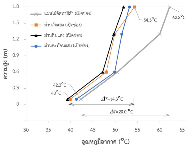
รูปที่ 5 อุณหภูมิอากาศที่ระยะความสูงต่าง ๆ ในปล่องระบายอากาศ (Air temperature at different heights in the ventilation chimney)
