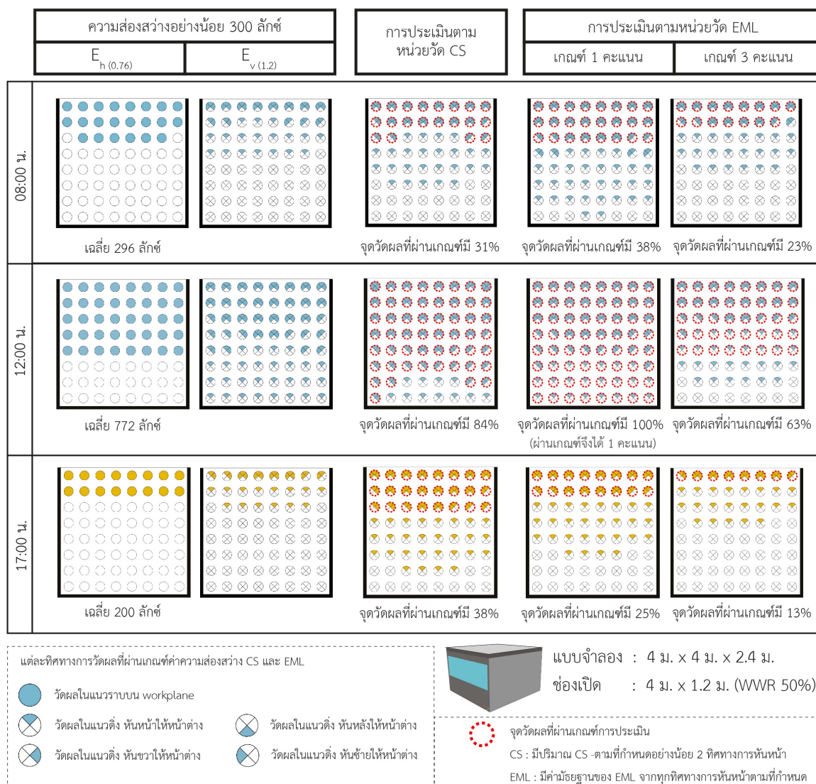
รูปที่ 3 แสดงแผนผังแบบจำลองที่ประเมินแสงในหน่วยวัด E_h(0.76) CS และ EML ของช่วงเวลา 08:00 น. 12:00 น. และ 17:00 น (Evaluation of Measurement E_h(0.76) , CS and EML in 8 A.M., 12 A.M. and 5 P.M.).
