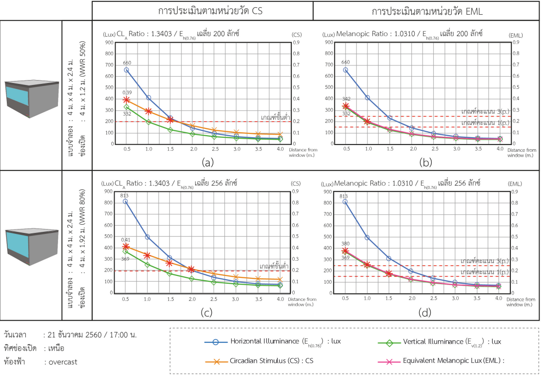
รูปที่ 5 แผนภูมิแสดงปริมาณ E_{h(0.76)} E_{v(1.2)} CS และ EML ของแบบจำลองที่ช่องเปิดมีอัตราส่วนพื้นที่ช่องเปิดต่อพื้นที่ผนังที่ร้อยละ 50 และ 80 (Measurement of E_{h(0.76)} E_{v(1.2)} CS and EML in WWR50% and WWR80% Model)
