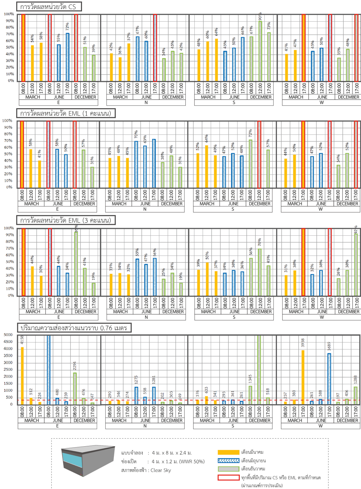
รูปที่ 7 แสดงแผนภูมิร้อยละพื้นที่ที่ผ่านเกณฑ์การประเมินแสงสำหรับหน่วยวัด Eh(0.76), CS และ EML ในแต่ละทิศทางช่องเปิด (Percentage of Passing Area a Criterion of Evaluation of Measurement Eh(0.76), CS and EML in All Direction of Window)
