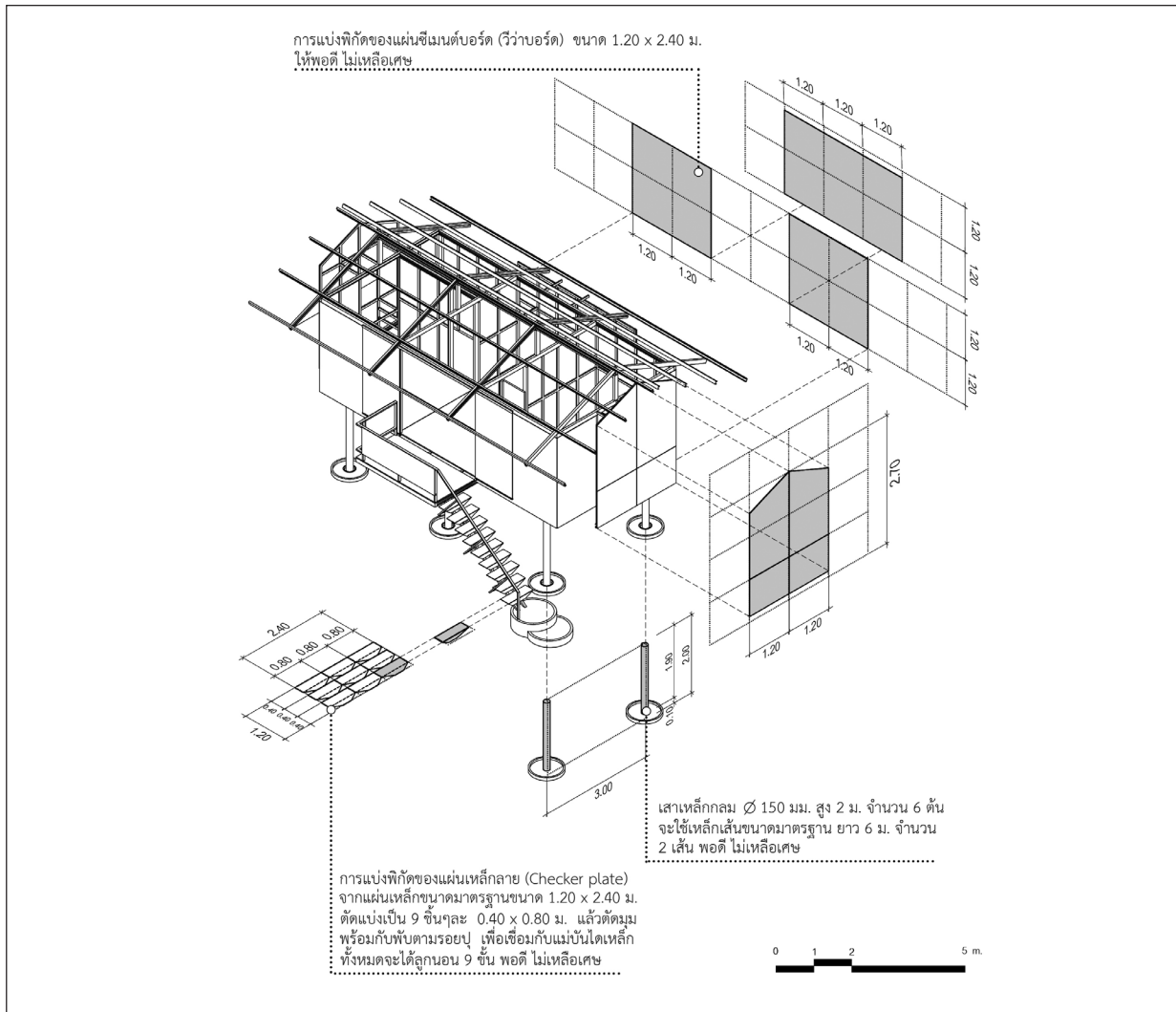
ที่มา: by author รูปที่ 7 ตัวอย่างภาพวิเคราะห์ประสิทธิภาพอาคาร ด้านการใช้ทรัพยากรวัสดุก่อสร้างอย่างประหยัด ลงตัวไม่เหลือเศษ ของกรณีศึกษาโครงการบ้านพอตดี้ ออกแบบโดย สถาปนิก สุริยะ อัมพันศิริรัตน์ บ. Walllasia จำกัด (Example of analysis in building performance in term of saving construction materials resource; efficiently building without scrap, from the case study of Baan Pordee Pordee, designed by architect Suriya Umpansiriratan, Walllasia.)
