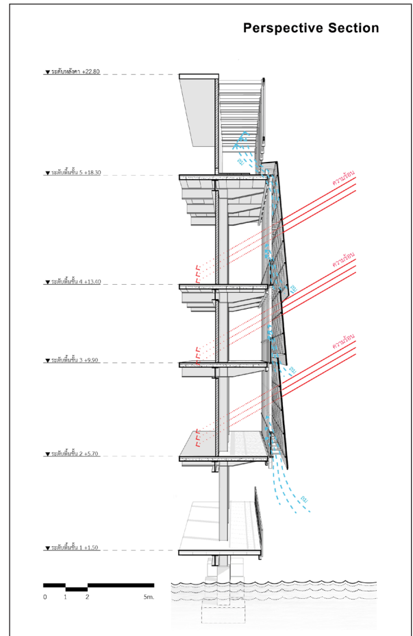
ที่มา: by author รูปที่ 6 ตัวอย่างภาพวิเคราะห์ประสิทธิภาพอาคาร ด้านการป้องกันความร้อนและระบายอากาศของเปลือกอาคารกรณีศึกษาโครงการ Flagship Building มหาวิทยาลัยศิลปากร ออกแบบโดย บ. Geodesic Design จำกัด (Example of analysis in building performance in terms of energy saving; solar radiation protection and natural ventilation, from the case study of Flagship Building at Silpakorn University, designed by Geodesic Design.)
