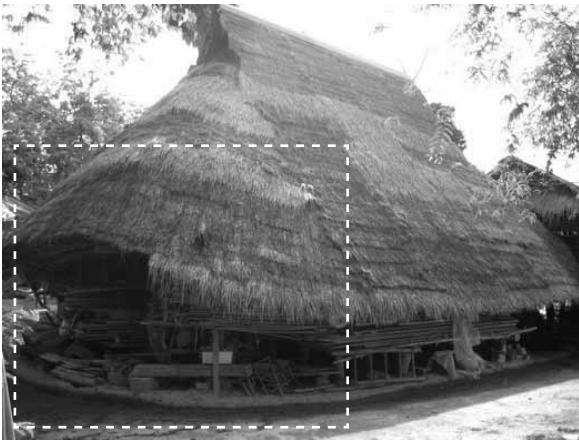
รูปที่ 16 การจัดฝังเสาตูปบริเวณกว้านที่สอบเข้าเพื่อให้อับกับโค้งหลังคาและฝังเรือนที่เรือนกระตองเต่าดั้งเดิมที่บ้านแม่ประจันต์
