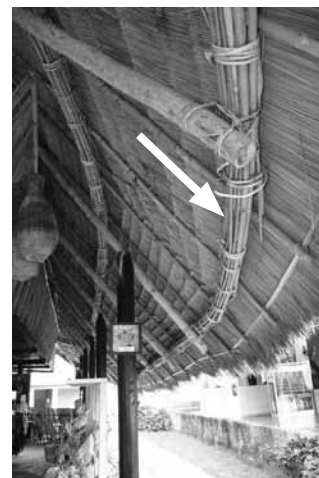
รูปที่ 15 กวางตูปที่เรือนจำลองที่ศูนย์วัฒนธรรมไทยทรงดำ (บ้านวัง) (ก) บริเวณชานหรือกว้าน (ข) บริเวณชายคา ด้านข้าง
