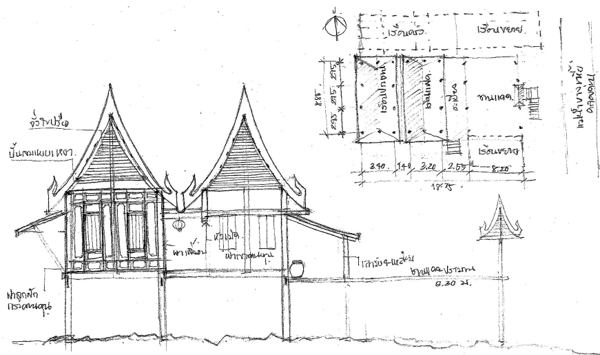
ภาพที่ 1 แสดงการสำรวจด้วยภาพวาด เรือนนายเซ่ง (จางเหยวียนเซ่ง) ที่มา: คณะผู้วิจัย
