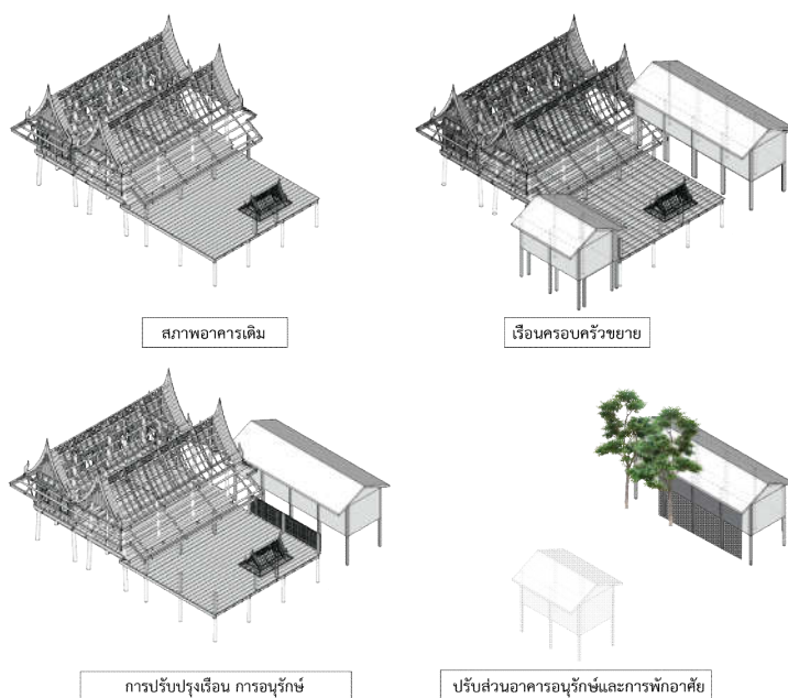
ภาพที่ 5 แสดงภาพจำลองเรือนด้วยโปรแกรมสร้างแบบ แนวทางการอนุรักษ์และบูรณะเรือนนายเซ่ง (จากเหวียนเซ่ง) ที่มา: คณะผู้วิจัย
