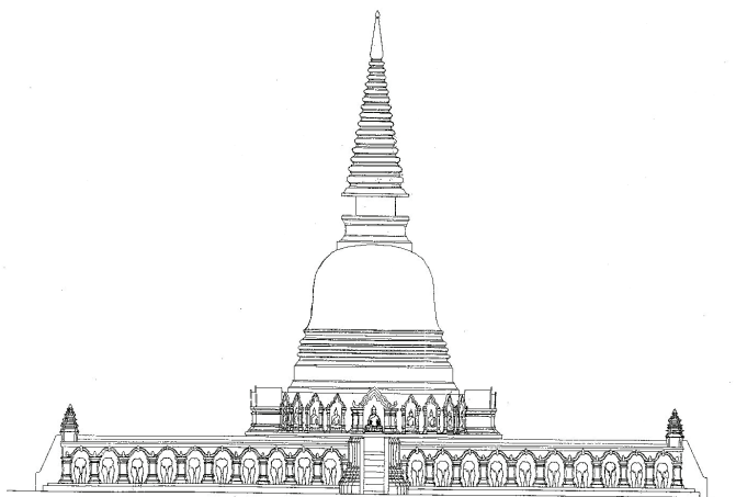
แผนผัง 2 รูปด้านเจดีย์ประธานวัดมเหยงคณ์ จังหวัดพระนครศรีอยุธยา
