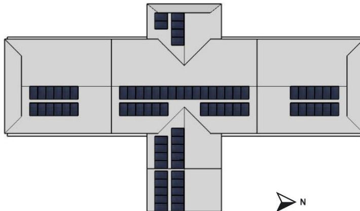
ภาพที่ 5 การติดตั้งแผงเซลล์แสงอาทิตย์บนอาคารหลังปรับปรุงแนวทางที่ 4
