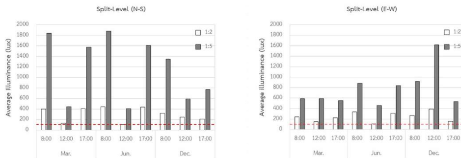
ภาพที่ 8 ผลการจำลองค่าความส่องสว่างแนวระนาบเฉลี่ย (ลักซ์) ที่ระดับ 1.50 เมตร จากพื้นชั้น 1 และ 1 ½ ของอาคารกรณีศึกษาแบบพื้นเล่นระดับ
