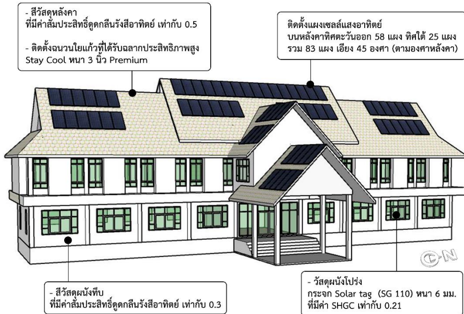
ภาพที่ 6 แบบร่างสามมิติอาคารกรณีศึกษาหลังปรับปรุง
