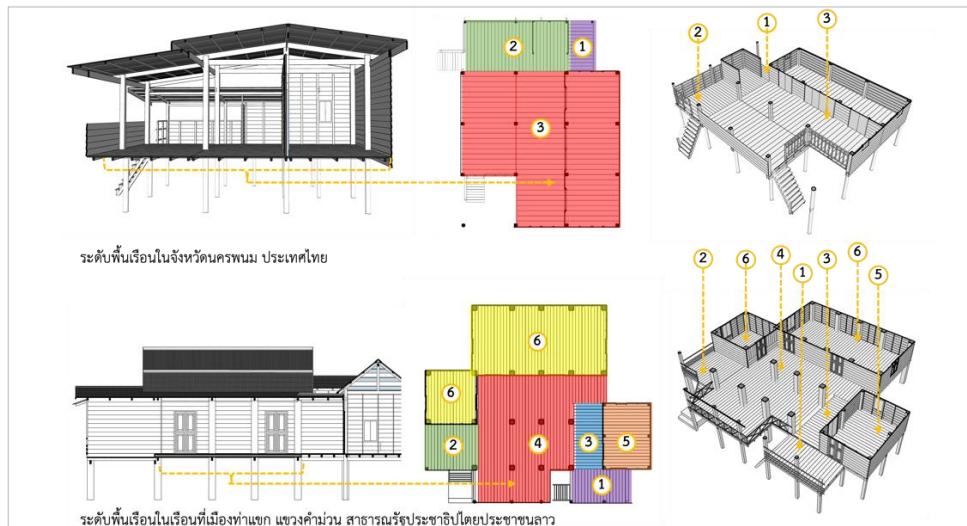
ภาพที่ 9 แสดงการเปรียบเทียบระดับพื้นเรือนที่มีความต่างกัน ใน เรือนผู้พูดภาษาแสมในจังหวัดนครพนมและเรือนที่เมืองท่าแขก แขวงคำม่วน สาธารณรัฐประชาธิปไตยประชาชนลาว
