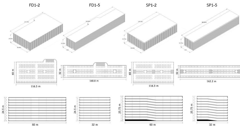
ภาพที่ 4 รูปแบบอาคารกรณีศึกษา (บน) ภาพไอโซเมตริก (กลาง)
