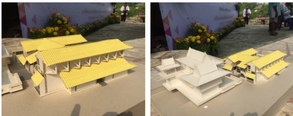
ภาพที่ 7 หุ่นจำลองศูนย์ฟื้นฟูและพัฒนาศักยภาพคนไร้บ้าน จ. ปทุมธานี โดยหน่วยงานภาครัฐที่พัฒนาเสร็จสิ้นแล้วก่อนนำไปก่อสร้าง
