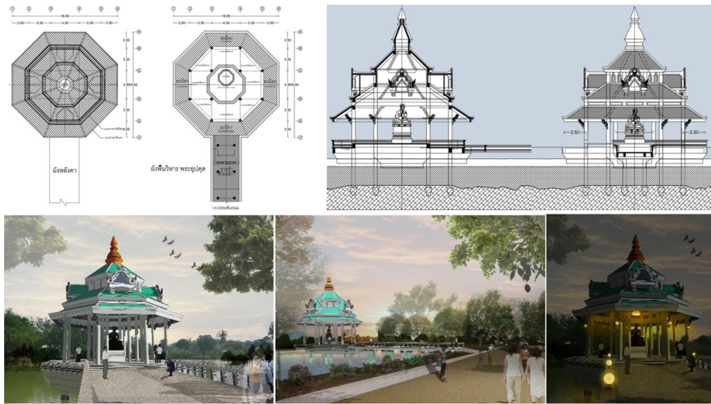
ภาพที่ 5 ผังหลังคา ผังพื้น รูปตัดและรูปด้านหน้าวิหาร (บน) และทัศนียภาพภายนอกวิหาร (ล่าง) ที่มา: ผู้นิพนธ์
