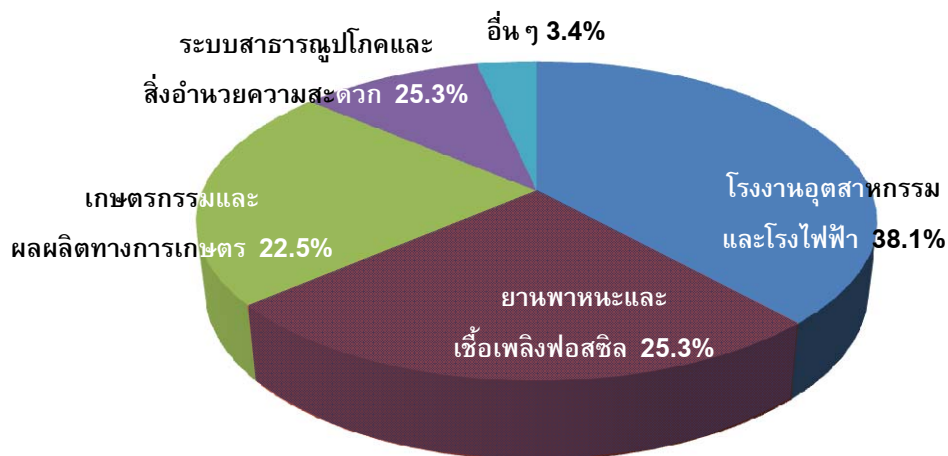
ภาพที่ 3 แผนภูมิแสดงสัดส่วนการปล่อยก๊าซเรือนกระจก (ที่มา : www.seed.slb.com )
