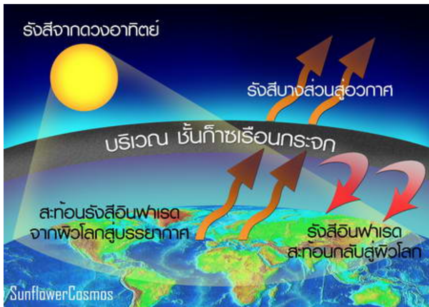
ภาพที่ 1 การเกิดปรากฏการณ์เรือนกระจก (ที่มา : http://sunflowercosmos.org )
