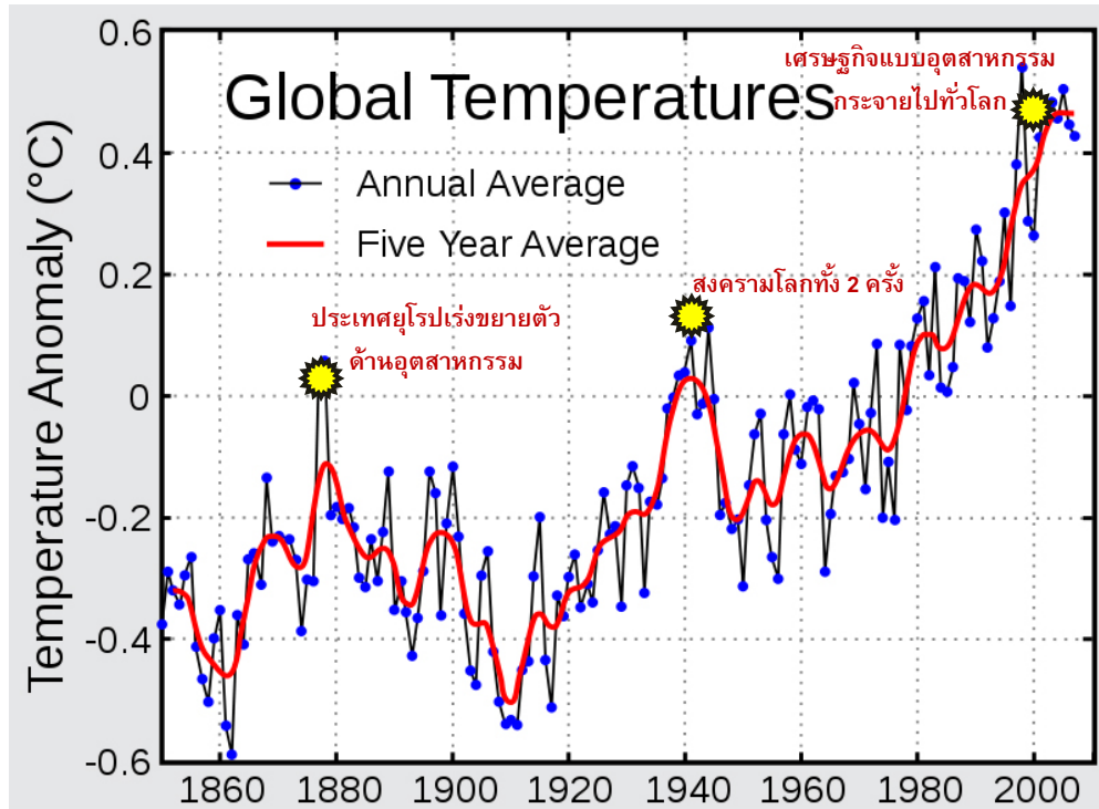
ภาพที่ 2 แผนภูมิแสดงระดับอุณหภูมิโลกโดยมหาวิทยาลัย อีสต์ แองเกลีย (ที่มา : www.seed.slb.com )
